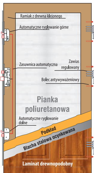
Profil skrzydła
