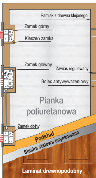
Profil skrzydła
