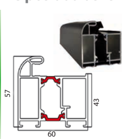
Ościeżnica TERMO
