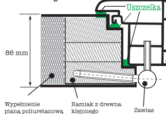
Profil skrzydła
