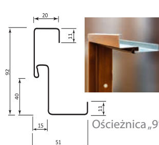
Ościeżnica „11”
