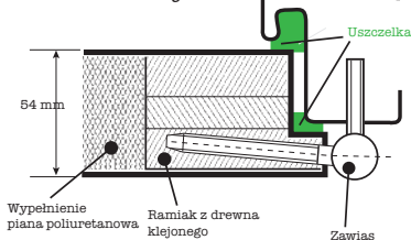
Profil skrzydła
