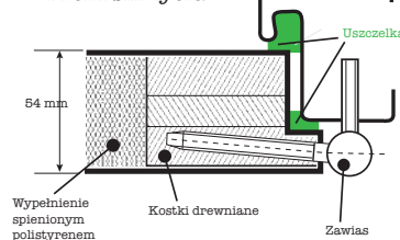
Profil skrzydła
