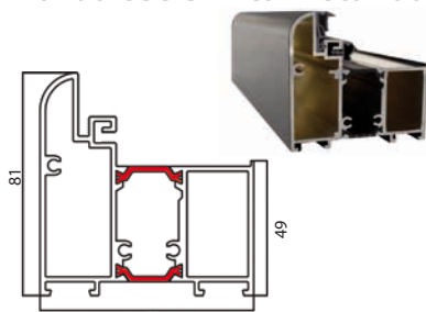
Ościeżnica TERMO PRESTIGE
