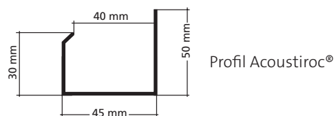
Profil C Acoustiroc®
