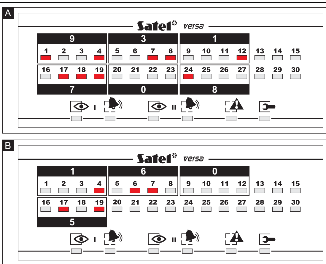
Rys. 4. Przykłady prezentowania wartości dziesiętnych przy pomocy diod LED w manipulatorze LED. W przykładzie A zaprogramowana jest wartość 931708, a w przykładzie B – 1605.
