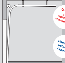
Nadproże Wysokie H (sprężyny skrętne z przodu)
