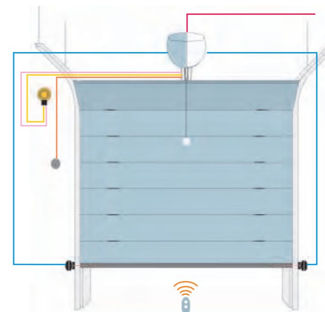
Schemat instalacji napędu SPIN
