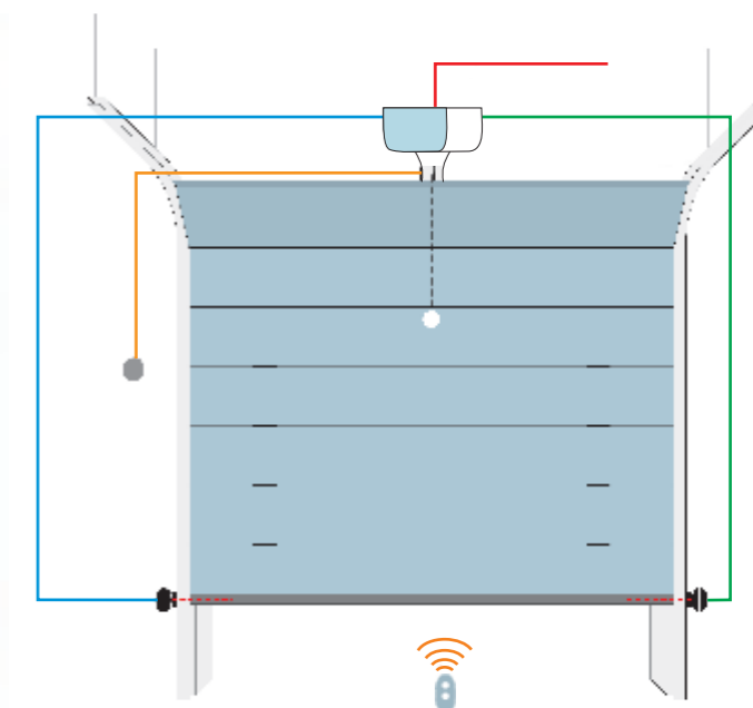
Schemat instalacji napędu Shel
